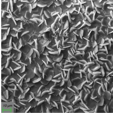
SURFACOTE 125, 500fache Vergrößerung
