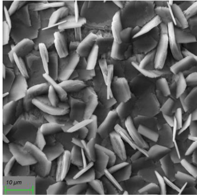
SURFACOTE 125, 1000fache Vergrößerung
